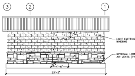
4 SIDE ELEVATION SCALE: 1/4" = 1'-0"
