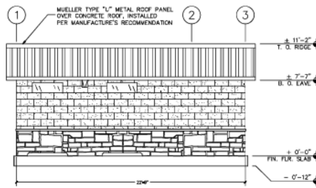
2 SIDE ELEVATION SCALE: 1/4" = 1'-0"
