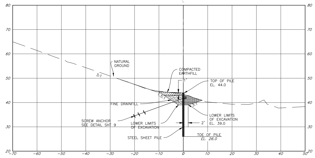
STA. 170+20
