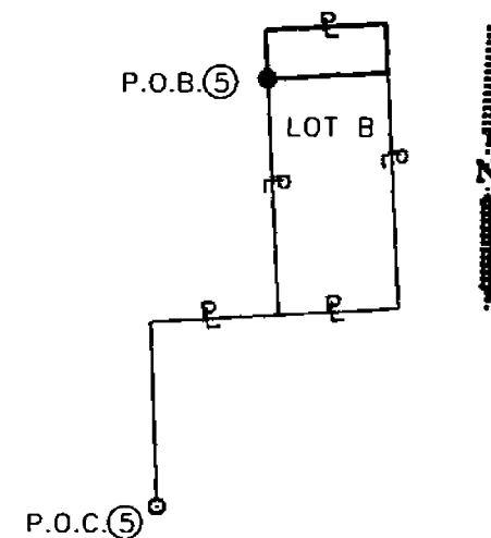
PARENT TRACT INSET PARCEL 5 N.T.S.
