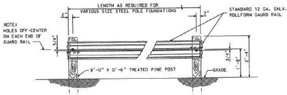
ELEVATION
